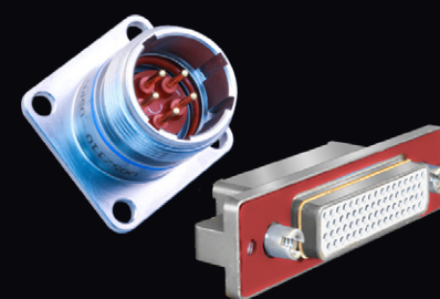
ThermaRex HT 耐熱コネクタ 高温300℃
