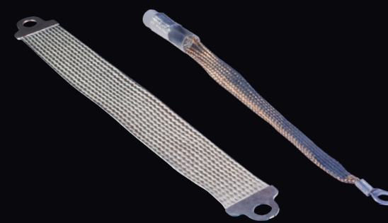
グランドストラップ・ 熱収縮スリーブ編組シールド付き 軽量/柔軟特性 ArmorLite™
