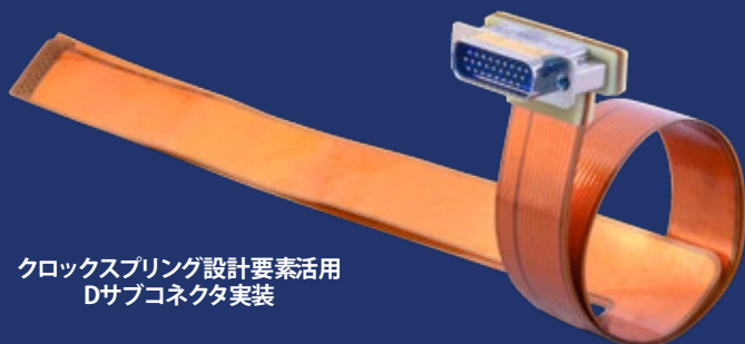
振動・衝撃耐性 リジッドFPC複合組立品 Mighty Mouse – Micro-D – RF ケーブル
