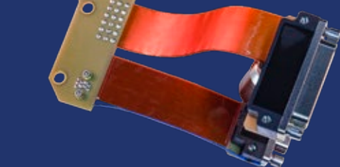
2段重ね結合 Micro-Dコネクタ 実装
