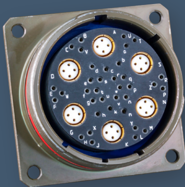
SuperNine® 高速通信・差動伝送
