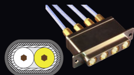
ウルトラTWINAXコンタクト用 整合インピーダンス ツイストペア ケーブル
