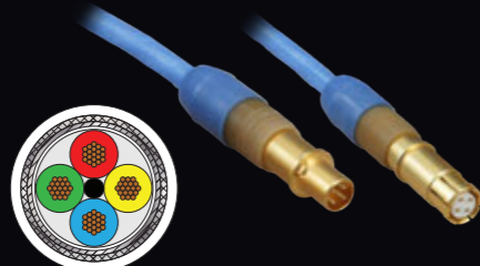
QUADRAXコンタクト用 航空宇宙グレードクアドケーブル
