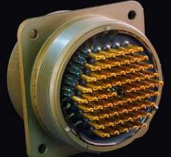
MIL-DTL-5015 シリーズIII
