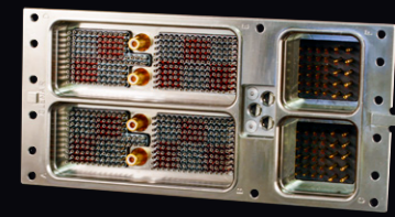
ARINC 600 サイズ1~3 EMIフィルター内蔵
