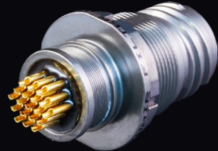
Mighty Mouse 805シリーズ ジャムナットレセプタクル 半田カップ
