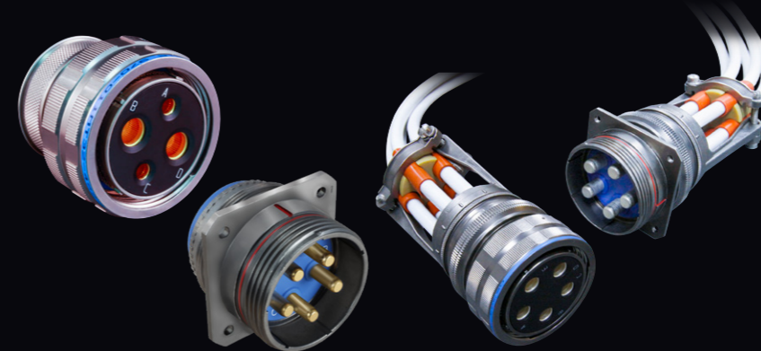
高密度・高度特性を持つ PowerTrip™ コネクタ 5015由来電源インサート配列 + 38999由来三条ネジ嵌合 + 28840由来堅牢ネジ より高い定格電流・First-Make Last-Mate技術・ EMIフィルタ・ガラスハーメチック
