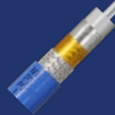
300サイズ 18GHz FEP被覆 3層編組
