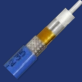
235サイズ 18GHz FEP・ETFE 被覆 3層編組
