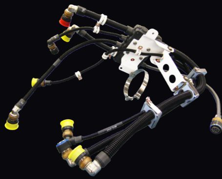
戦闘機用多分岐ハーネス
